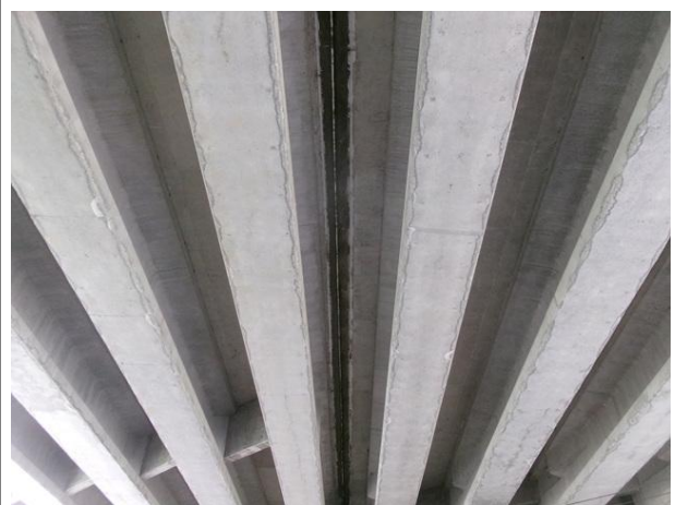
바닥판하면
